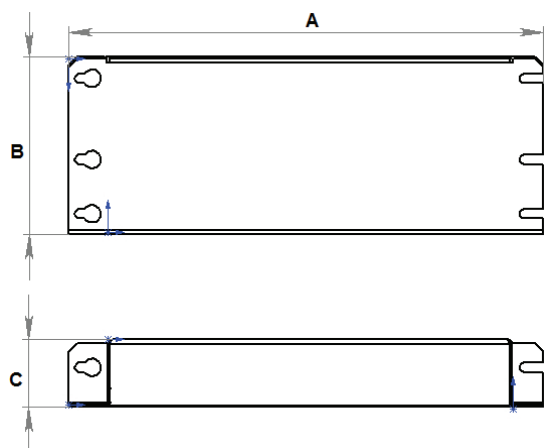
Рис. 1 Габаритно-присоединительные размеры фильтров
